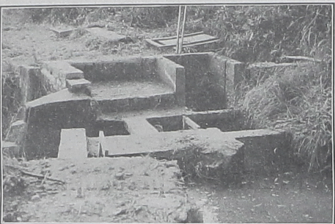
Trabalho de prevenção nas proximidades da Porcelana Schmidt
