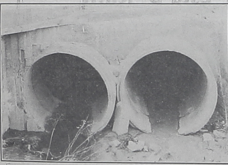
Na foto acima as manilhas antigas com apenas 80cm de diâmetro. Na foto abaixo as novas manilhas que já tem 2,20m
